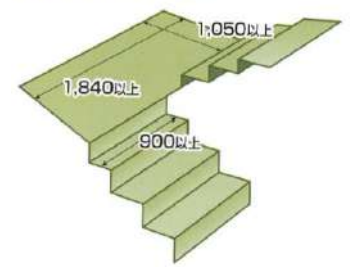
踊り場の許容寸法(mm)
